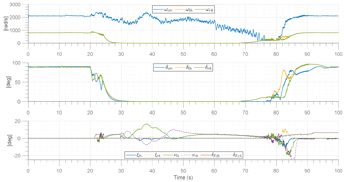
Fig. 15 Actuator Tracking
